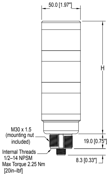
Abbildung 2. Abmessungen der Modelle Compact und Beacon
