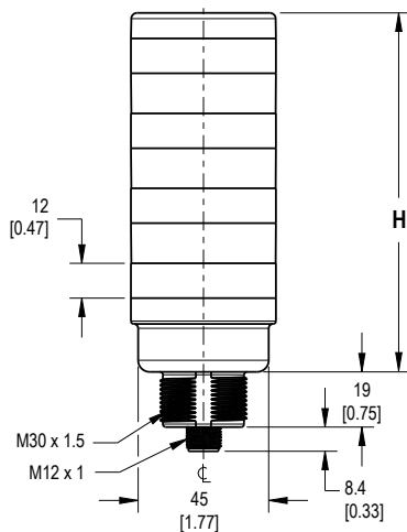
Abbildung 2. Abmessungen der Modelle Compact und Beacon
