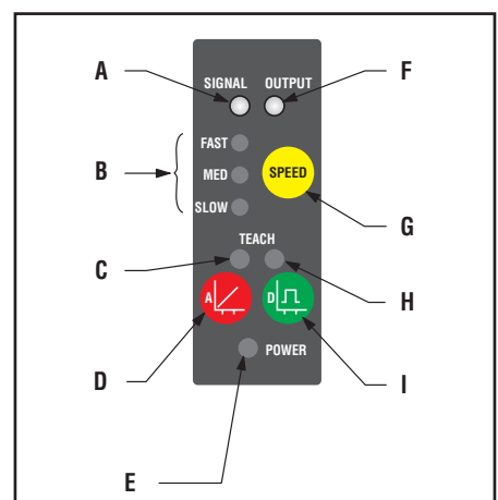
Abbildung 2. Merkmale des LT3-Entfernungsmessgeräts
