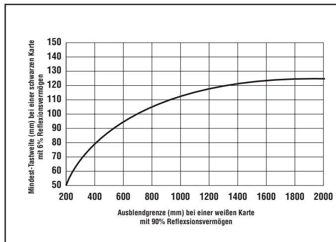
Abb. 11. Q60 – Verhältnis zwischen Mindest-Tastweite und eingestellter Ausblendgrenze
