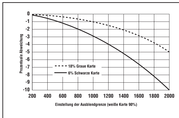
Abb. 10. Abweichung der Ausblendgrenze
