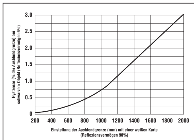
Abb. 12. Q60 – Hysterese
