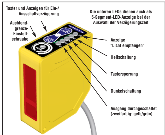
Abb. 1. Merkmale des Q60
