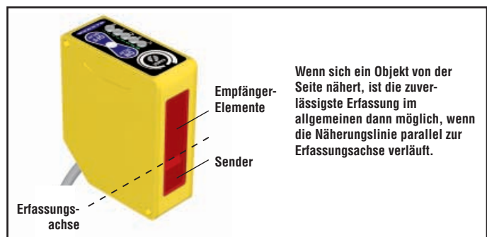
Abb. 3. Erfassungsachse des Q60
