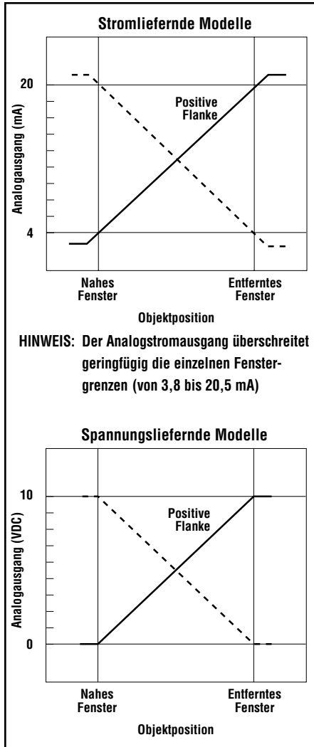
Abbildung 3. Ausgangsstrom als Funktion der Objektposition
