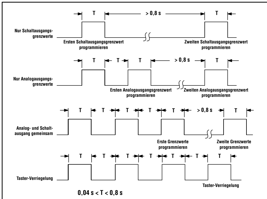
Abbildung 2. Zeitablaufprogramme für externe Programmierung (Remote TEACH)
