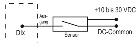
Es ist zu beachten, dass der Sensor und das SureCross-Gerät unter Umständen dieselbe Stromquelle haben müssen.
