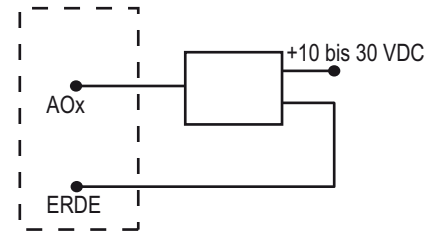
Dreileiter-Analogausgangsschaltgerät mit externer Versorgung (nicht vom DX80-Gerät).
