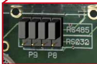
Kommunikationspins
