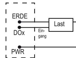
Anschlussdiagramm für einen Dreileiter-npn-Ausgang.
