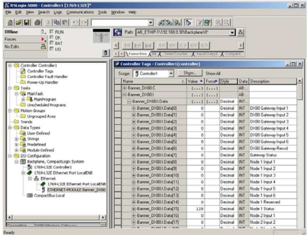
Banner-DX80-Eingänge von Funkvorrichtungen
