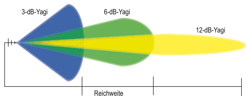
Mit zunehmender Verstärkung der Yagi-Antenne wird das Funksignal entlang eines bestimmten Wegs stärker fokussiert.
