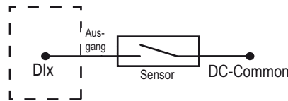
Es ist zu beachten, dass der Sensor und das SureCross-Gerät unter Umständen dieselbe Stromquelle haben müssen.
