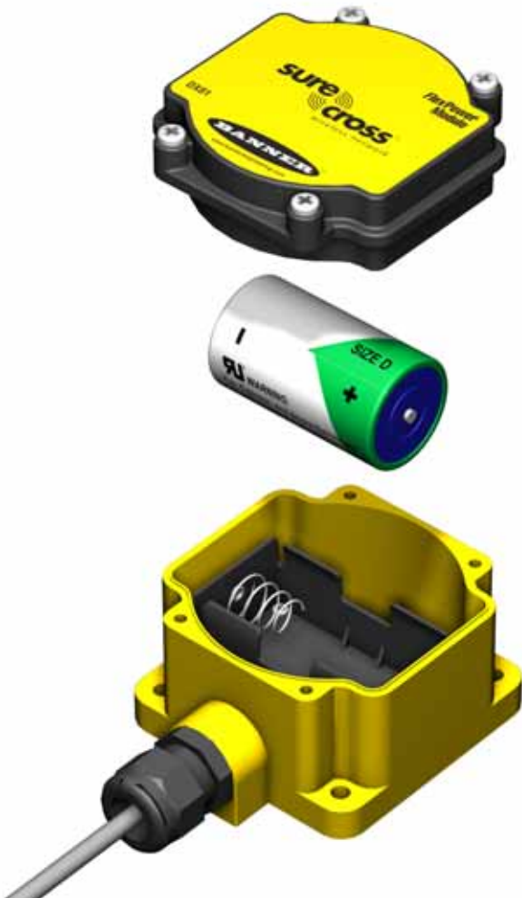
DX81-Batterieaustausch
