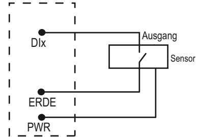
Anschlussdiagramm für einen Dreileiter-npn-Sensor mit Versorgung über den Klemmenblock des DX80-Geräts.
