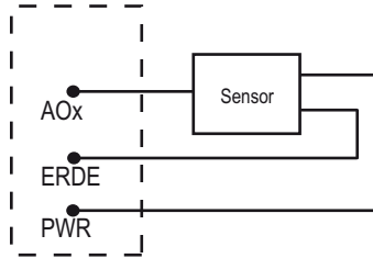
Dreileiter-Analogausgangsschaltgerät mit Versorgung vom DX80-Gerät.
