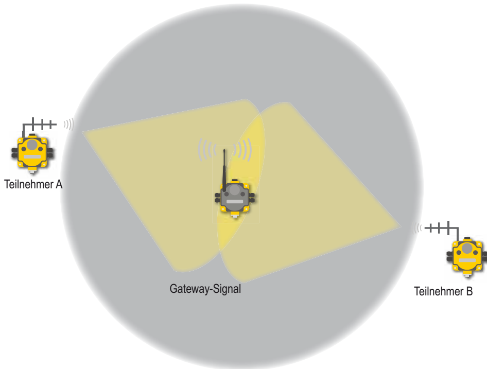
Eine Yagi-Antenne strahlt ein Signal in einer Richtung ab.
