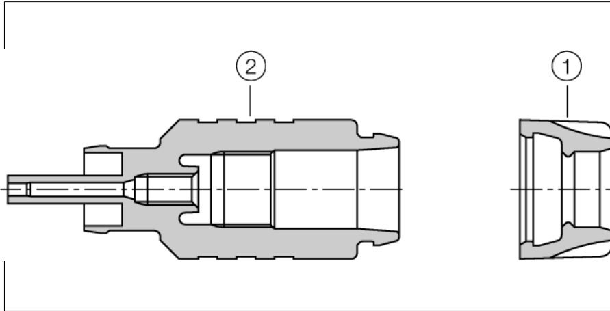
可现场接线的IP-Link光纤公头
