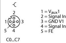
M12 × 1 Input
