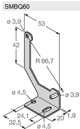
SMBQ60 3067592 ángulo de montaje, acero inoxidable, para modelo Q60
