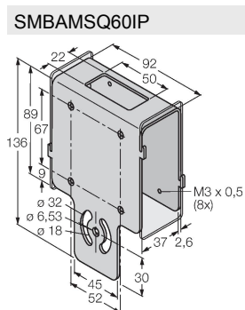
SMBAMSQ60IP 3073441 carcasa de protección con cristal protector, acero inoxidable, para modelo Q60
