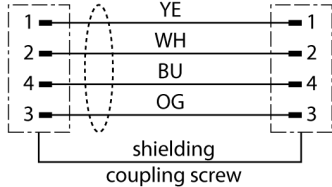
diagrama de conexiones
