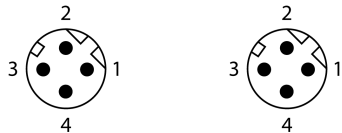
diagrama de conexiones
