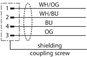
schéma de connexions
