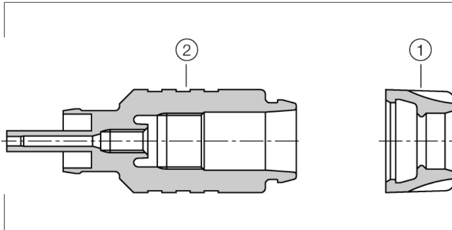
Connecteur mâle confectionnable pour fibre optique IP-Link
