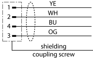
schéma de connexions
