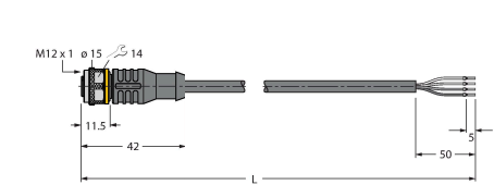
Rysunek wymiarowy Typ RKC4.4T-2/TEL Nr kat. 6625013
