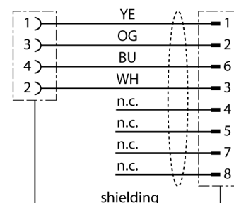
schemat obwodu
