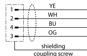
schemat obwodu
