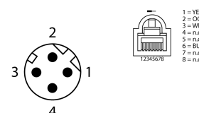
schemat obwodu
