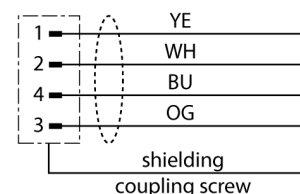
schemat obwodu
