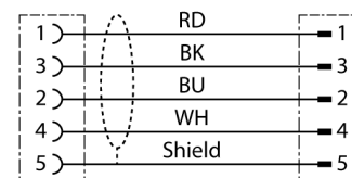
schemat obwodu
