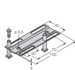
Șină de montaj pentru carcase rectangulare CK/CP40; material: VA 1.4301
