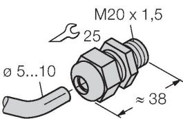
Presetupă M20 × 1.5
