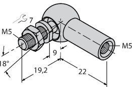
Cuplaj articulat pentru element de poziționare ghidat, oțel inoxidabil
