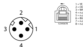
Schema de conexiuni
