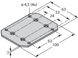
Монтажная пластина для расходомера FTCL для монтажа спереди
