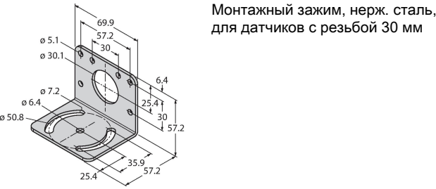
SMB30MM 3027162
