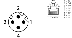
Devre şeması
